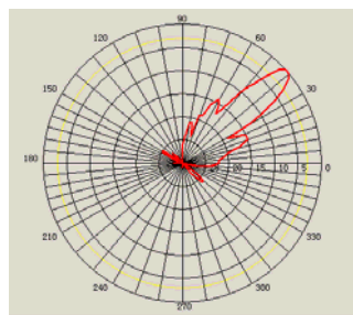
H-plane
