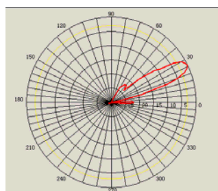
E-plane
